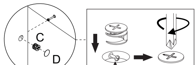
Detalhe 5 Detail/Detalle
