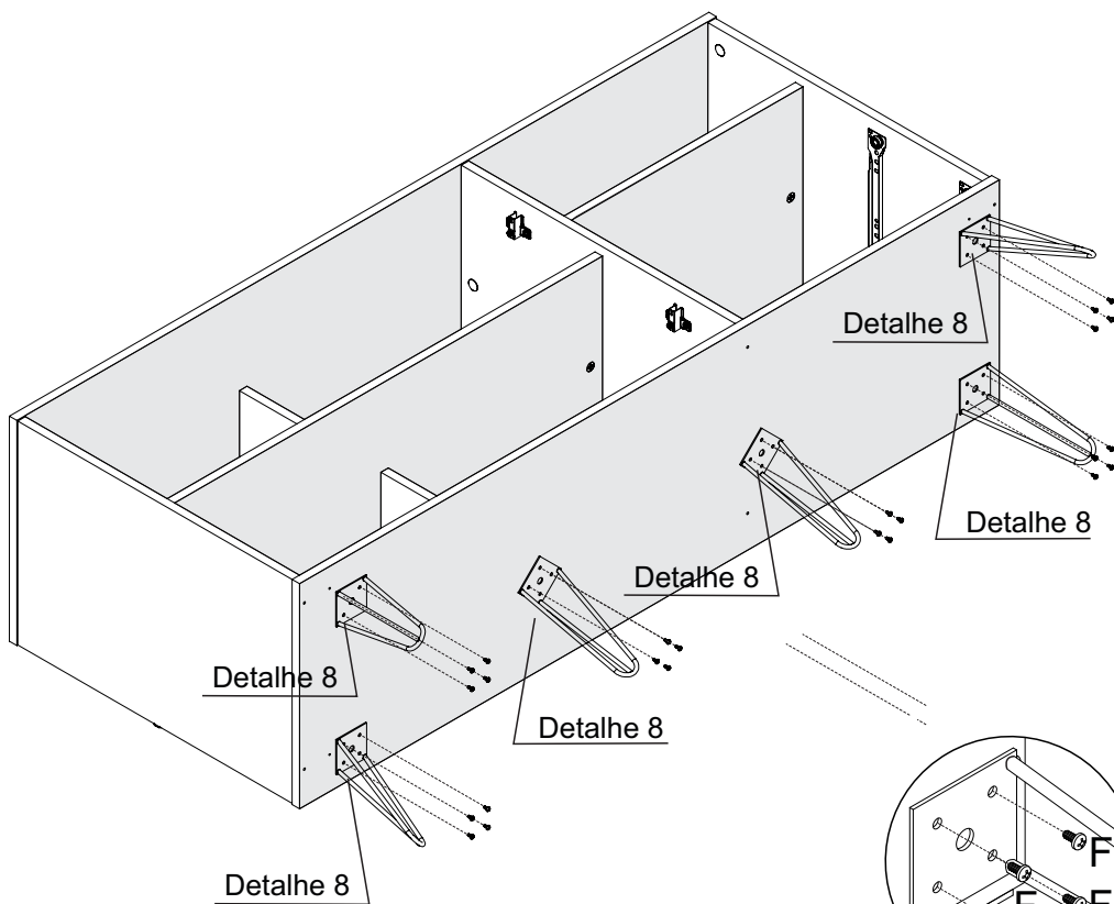
Detalhe 8 Detail/Detalle
